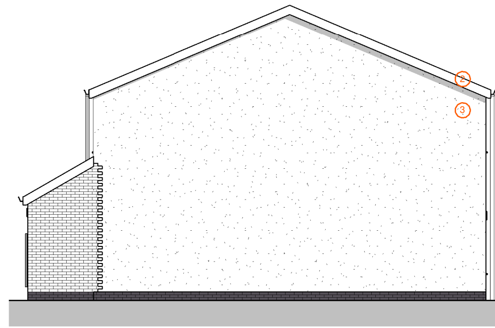
F1 Side Elevation 04 1 : 100
