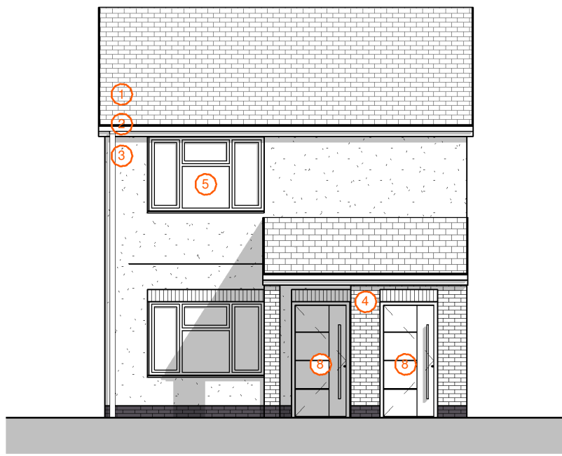
F1 Front Elevation 01 1 : 100
